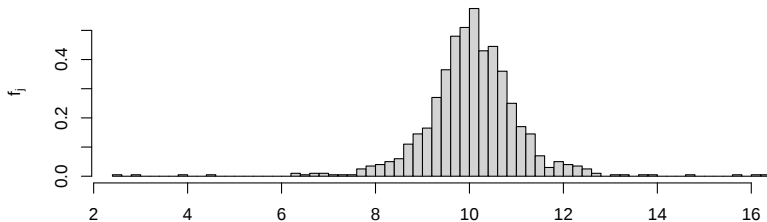
Merkmal mit großer empirischer Kurtosis (12.188)
