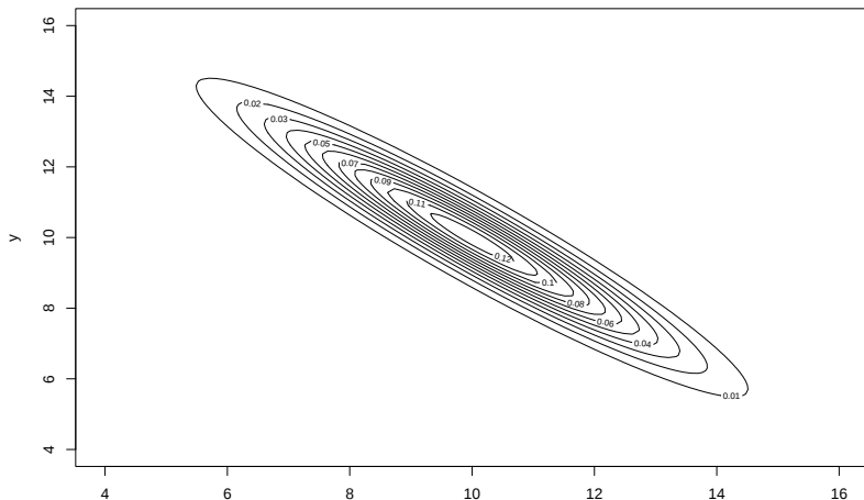
Isophöhenlinien der mehrdimensionalen Normalverteilungsdichte
