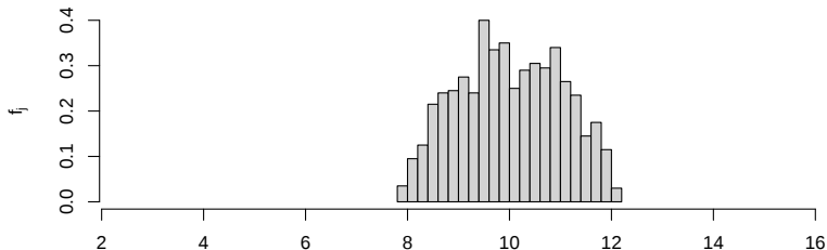
Merkmal mit kleiner empirischer Kurtosis (2.088)
