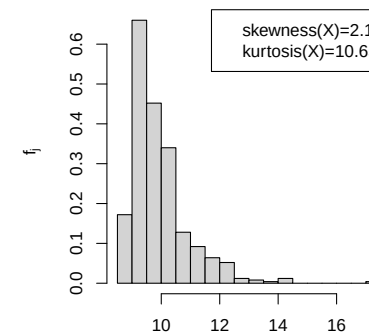
Linkssteil mit großer emp. Kurtosis
